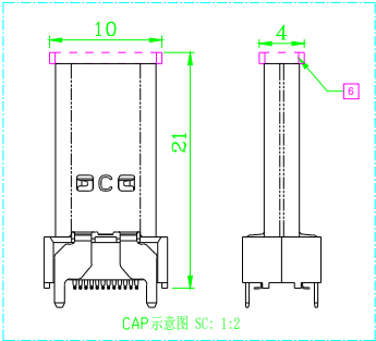
CAP 示意图 SC: 1:2
